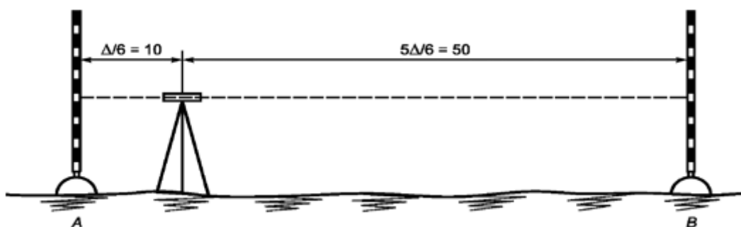
Amplasarea nivelmetrului și mirelor pentru a doua serie de măsurări
